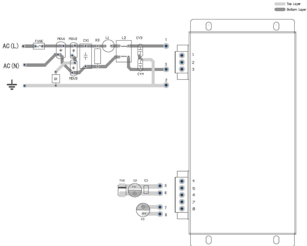
图 3： EMC 推荐电路 PCB 布板图
