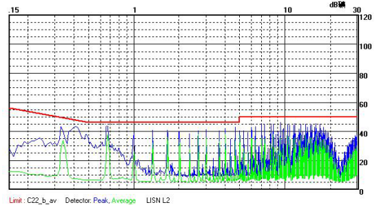
URF4812P-6WR2 传导骚扰 Class B 测试效果图 (负线)
