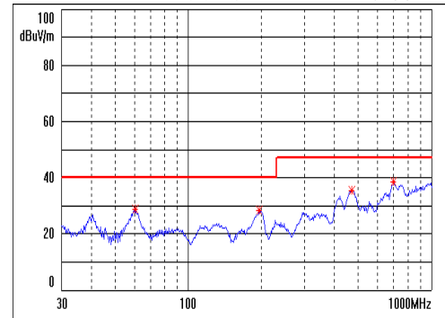
URF4812P-6WR2 辐射骚扰 Class B 测试效果图 (负线)
