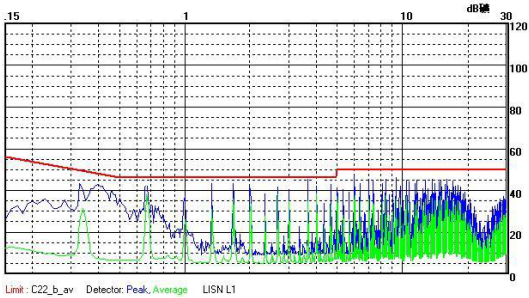
URF4812P-6WR2 传导骚扰 Class B 测试效果图 (正线)
