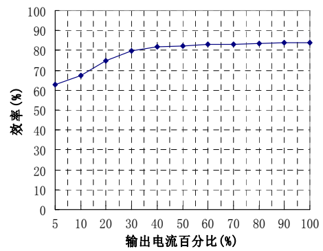
输出负载VS效率曲线图
