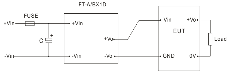
标称输入电压为 24V 时, C \geq 330\mu\text{F}/50\text{V} 标称输入电压为 48V 时, C \geq 330\mu\text{F}/100\text{V} FT-A/BX1D 为我司脉冲群抑制器, 具体型号请参照选型手册。 图 3
