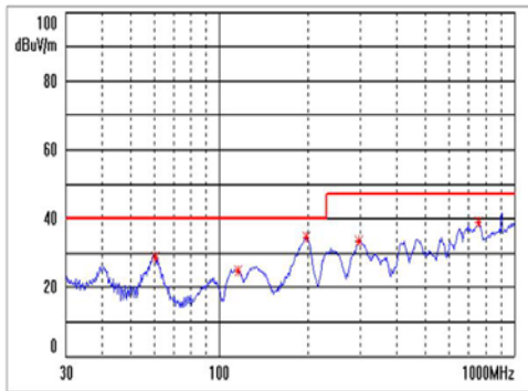
URF4812P-6WR2 辐射骚扰 Class B 测试效果图 (正线)
