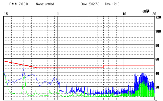
F2405S-2WR2 传导骚扰测试效果图 (负线)
