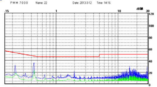
E2415S-2WR2 传导骚扰测试效果图 (负线)
