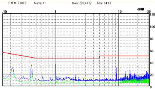
E2415S-2WR2 传导骚扰测试效果图 (正线)
