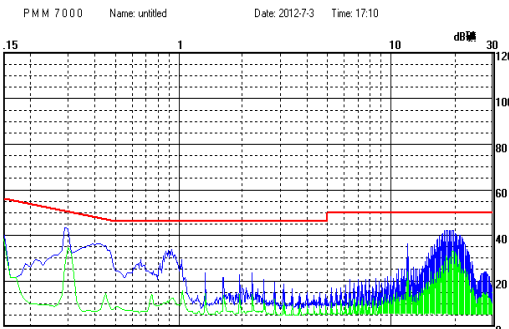
F2405S-2WR2 传导骚扰测试效果图 (正线)
