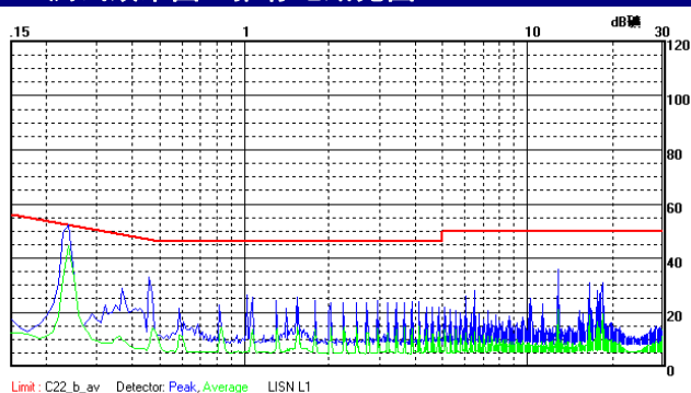
B0505M-2WR2 传导骚扰 Class B 测试效果图 (正线)
