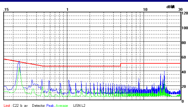
B0505M-2WR2 传导骚扰 Class B 测试效果图 (负线)
