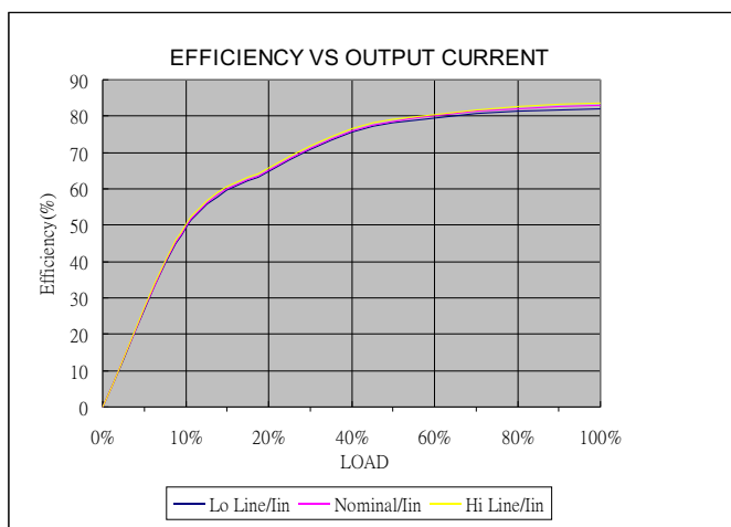
M1-0505SS2
