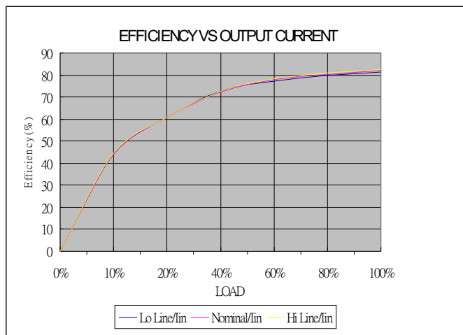
M1-2405SS2
