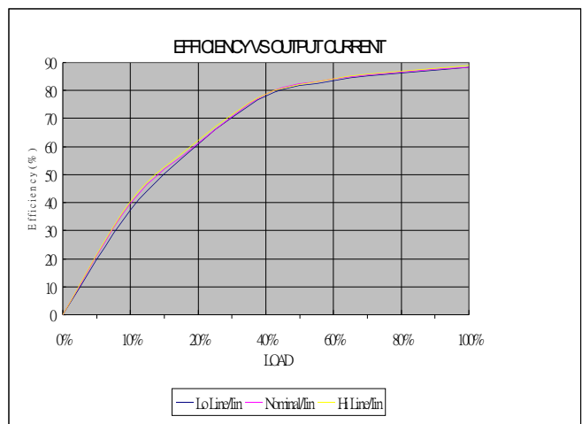
M1-2415S2
