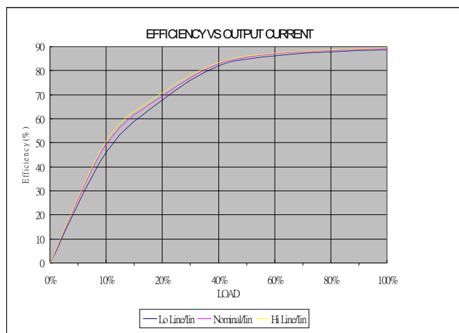
M1-0515S2
