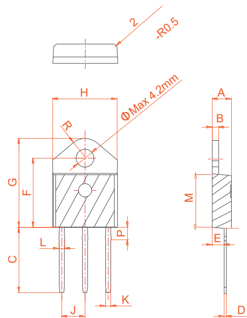
TO-3P Ins
