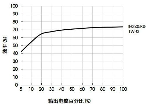
效率Vs输出负载 ( V_{in}=5\text{V} )
